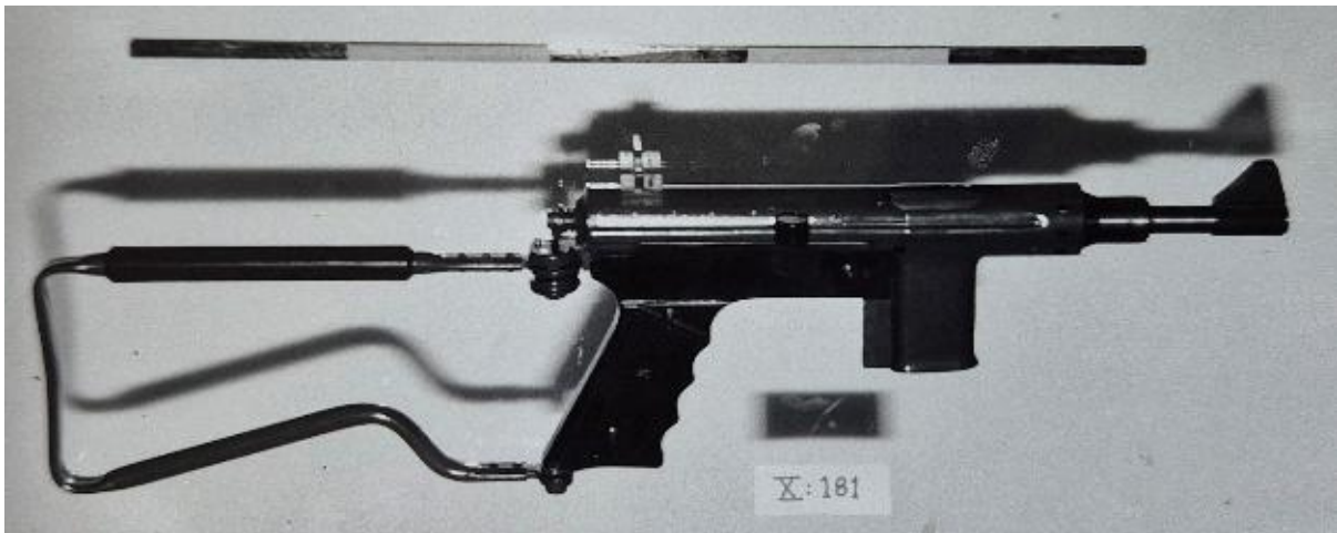
Lätt kulsprutepistol 67-74 W
